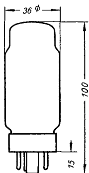
Kolbenabmessungen
