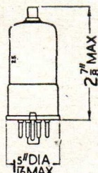
6K7GT.
