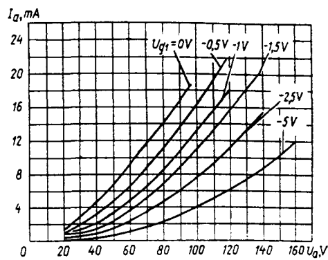
Усредненные анодные характеристики (триодное включение) U_h = 6,3 V
