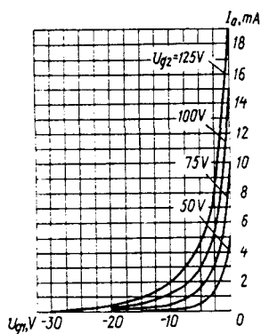
Усредненные анодно-сеточные характеристики U_h = 6,3 V, U_a = 250 V
