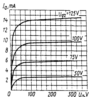
Усредненные анодные характеристики U_h = 6,3 В, U_{g1} = -1 В
