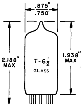
BASE 9 PIN BUTT JEDEC E9-1
