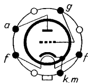
Sockelschaltsschema
