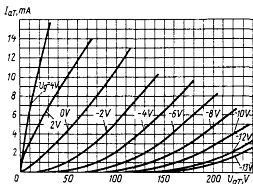
Усредненные анодные характеристики триода U_h = 6,3 В
