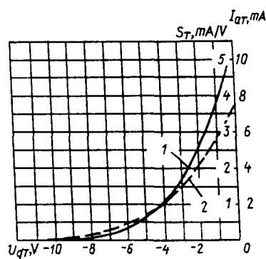
Усредненные характеристики триода: 1 — анодно-сеточные; 2 — крутизна U_h = 6,3 В, U_{aT} = 100 В
