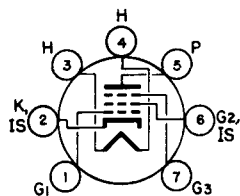
BASING DIAGRAM JEDEC 7EN
