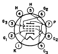
9NB
