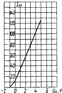
Усредненная начальная анодная характеристика (для одного диода) U_h = 6,3 \text{ V}, R_a = 40 \text{ k}\Omega
