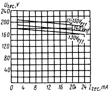
Усредненные характеристики выпрямленного напряжения в зависимости от выпрямленного тока U_h = 6,3 \text{ V}, R_a = 200 \Omega, C_{\text{filter}} = 8 \mu\text{F} Averaged characteristics of rectified voltage versus rectified current U_h = 6.3 \text{ V}, R_a = 200 \Omega, C_{\text{filter}} = 8 \mu\text{F}
