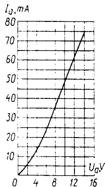
Усредненная анодная характеристика (для одного диода) U_h = 6,3 \text{ V}
