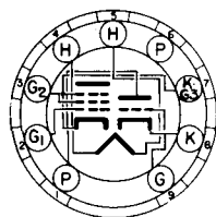
BOTTOM VIEW MINIATURE BUTTON 9 PIN BASE 9AE
