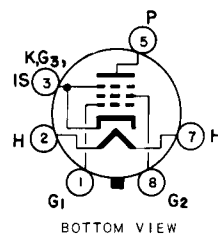
BASING DIAGRAM JEDEC 6CK
