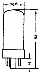
Kolbenabmessungen
