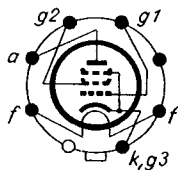
Sockelschaltschema
