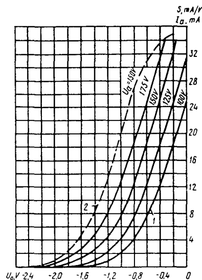
Усредненные анодно-сеточные характеристики триода: 1 — анодно-сеточные; 2 — крутизна характеристики U_h = 6,3 V Averaged anode-grid characteristics of triode: 1 — anode-grid; 2 — transconductance U_h = 6.3 V
