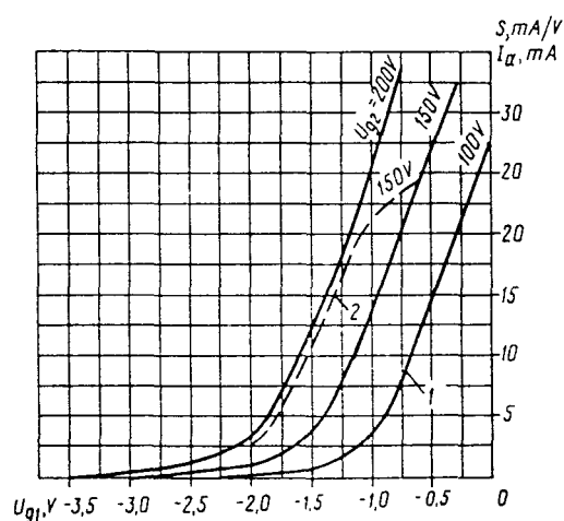
Усредненные анодно-сеточные характеристики пентода: 1 — ток анода; 2 — крутизна характеристики U_h = 6,3 V, U_a = 150 V Averaged anode-grid characteristics of pentode: 1 — anode current; 2 — transconductance U_h = 6.3 V, U_a = 150 V
