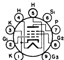
BASING DIAGRAM JEDEC 9AQ
