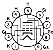
OTTOM VIEW BASING DIAGRAM JEDEC 9A0
