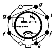
Sockelschaltschema
