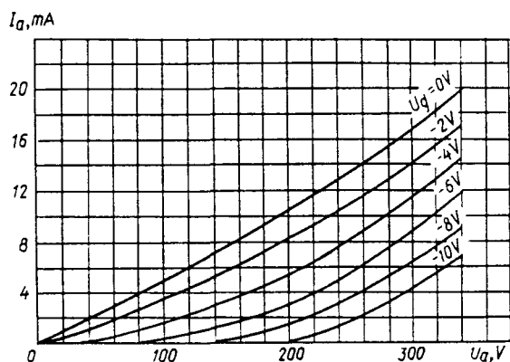
Усредненные анодные характеристики U_h = 6,3 \text{ V} , U_{a1} = 250 \text{ V}
