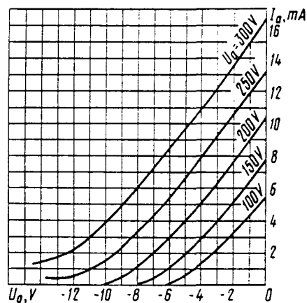
Усредненные анодно-сеточные характеристики U_h = 6,3 \text{ V} , U_{a1} = 250 \text{ V}
