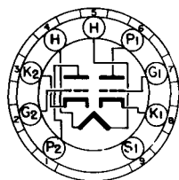
BOTTOM VIEW MINIATURE BUTTON 9 PIN BASE 9AU
