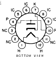
BASING DIAGRAM JEDEC 12BL
