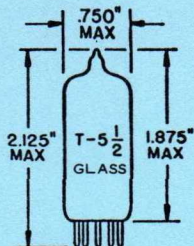
BASE 7 PIN MINIATURE BUTTON JEDEC E7-1
