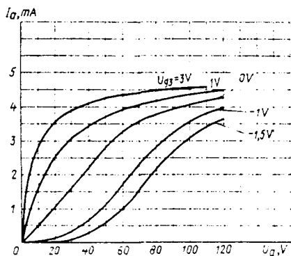
Усредненные анодные характеристики U_h = 6.3 \text{ V} , U_{g1} = 4 \text{ V} , U_{acc} = 75 \text{ V} Averaged anode characteristics: U_h = 6.3 \text{ V} , U_{g1} = 4 \text{ V} , U_{acc} = 75 \text{ V}
