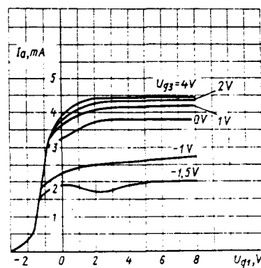
Усредненные анодно-сеточные характеристики U_h = 6.3 \text{ V} , U_a = 75 \text{ V} , U_{acc} = 75 \text{ V} Averaged anode-grid characteristics: U_h = 6.3 \text{ V} , U_a = 75 \text{ V} , U_{acc} = 75 \text{ V}
