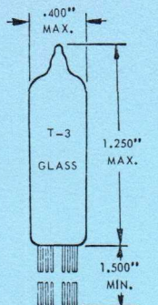
SUBMINIATURE BUTTON 8 FLEXIBLE LEADS JEDEC E8-10
