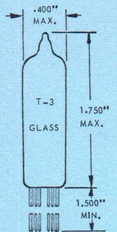
SUBMINIATURE BUTTON 8 FLEXIBLE LEADS JEDEC E8-10
