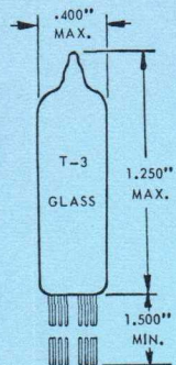
SUBMINIATURE BUTTON 8 FLEXIBLE LEADS JEDEC E8-10
