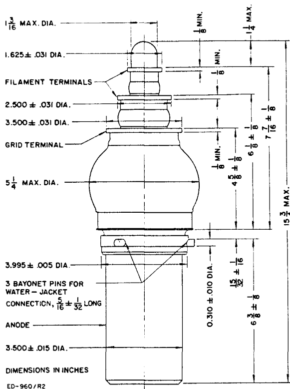
DIMENSIONS — ML-6426
