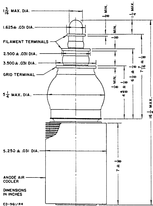
DIMENSIONS — ML-6427
