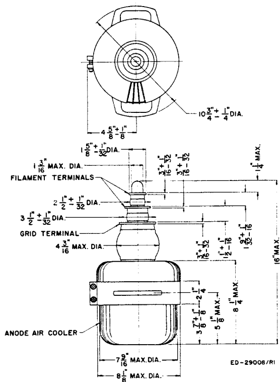
DIMENSIONS — ML-6425-F
