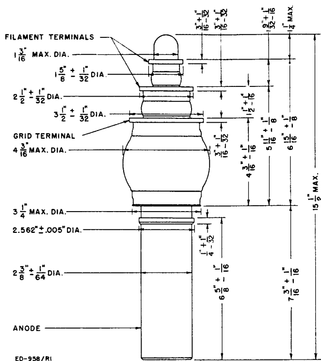
DIMENSIONS — ML-6424
