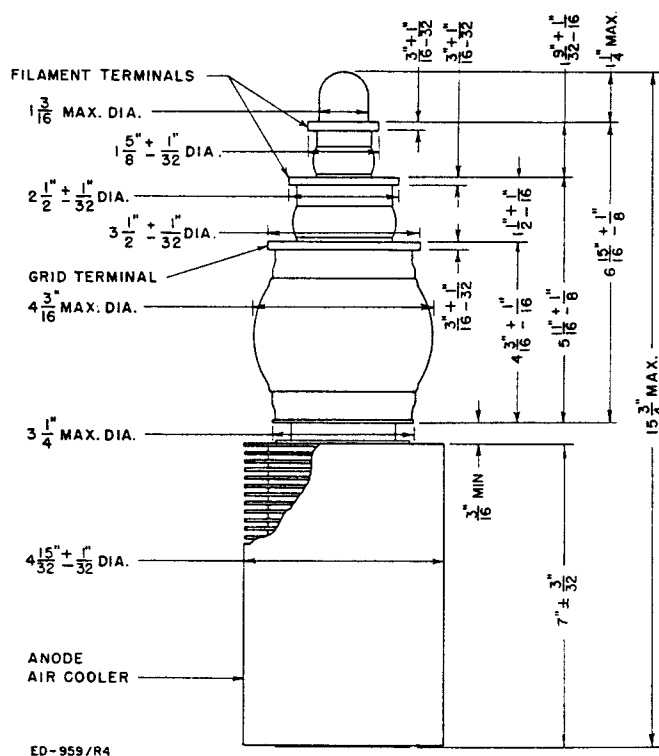
DIMENSIONS — ML-6425
