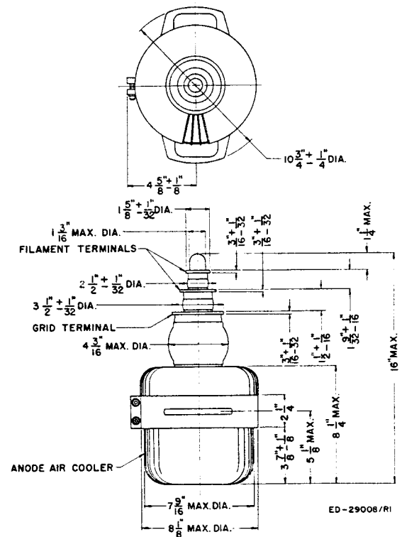
DIMENSIONS — ML-6425-F
