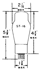
5Z3 - MEDIUM 4 PIN BASE
