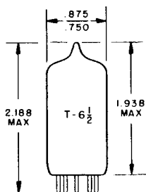
BASE 9 PIN BUTTON JEDEC E-9
