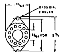
12 PRONG (DUODECAL)
