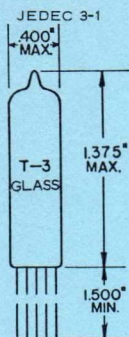
SUBMINIATURE BASE 8 PIN BUTTON JEDEC E8-10
