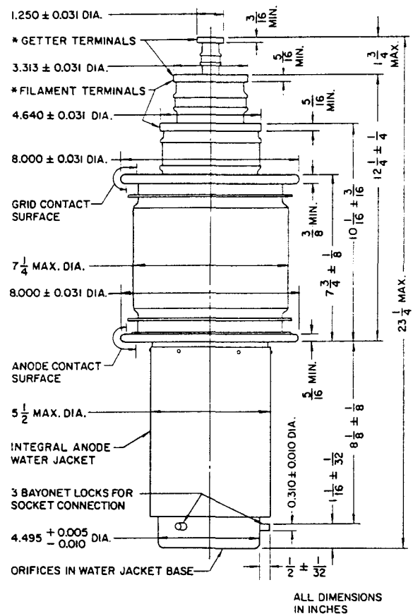
DIMENSIONS — ML-5682K
