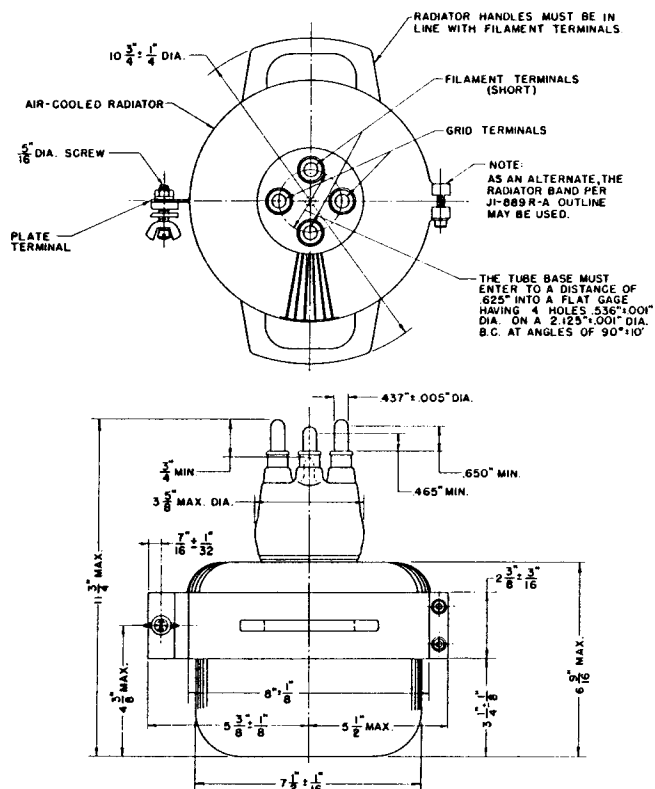
DIMENSIONS — ML-5667
