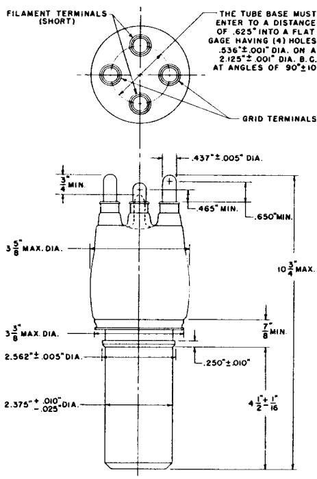
DIMENSIONS — ML-5666
