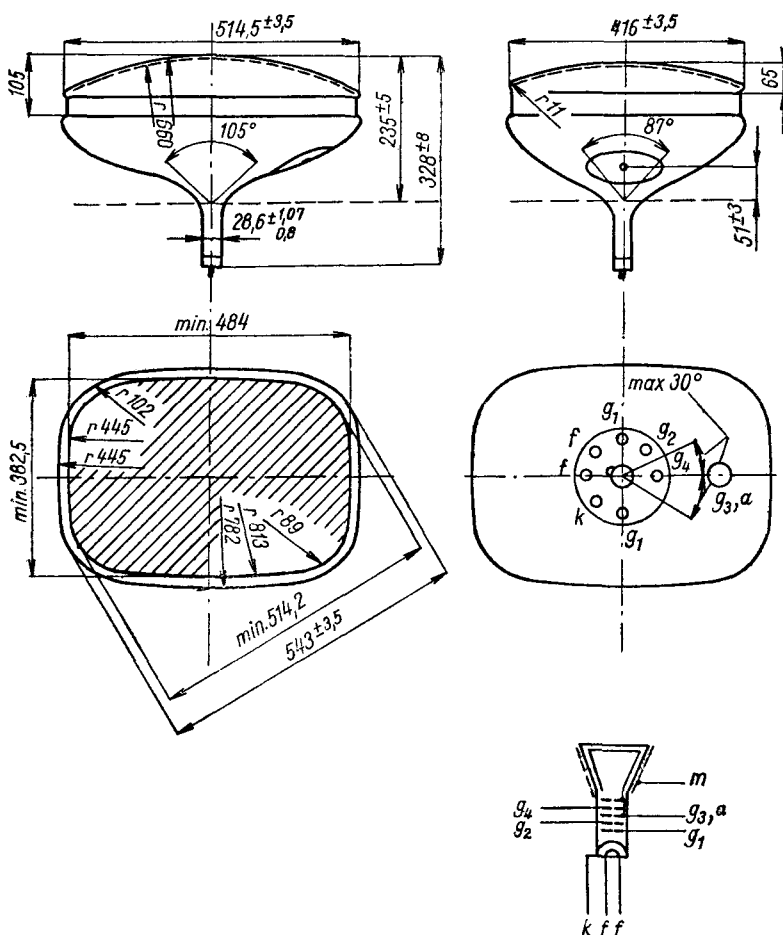
Obr. 149. Zapojení patice a rozměry obrazovky 531QQ44.
