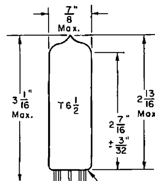
Miniature 9-Pin (JEDEC E9-1)
