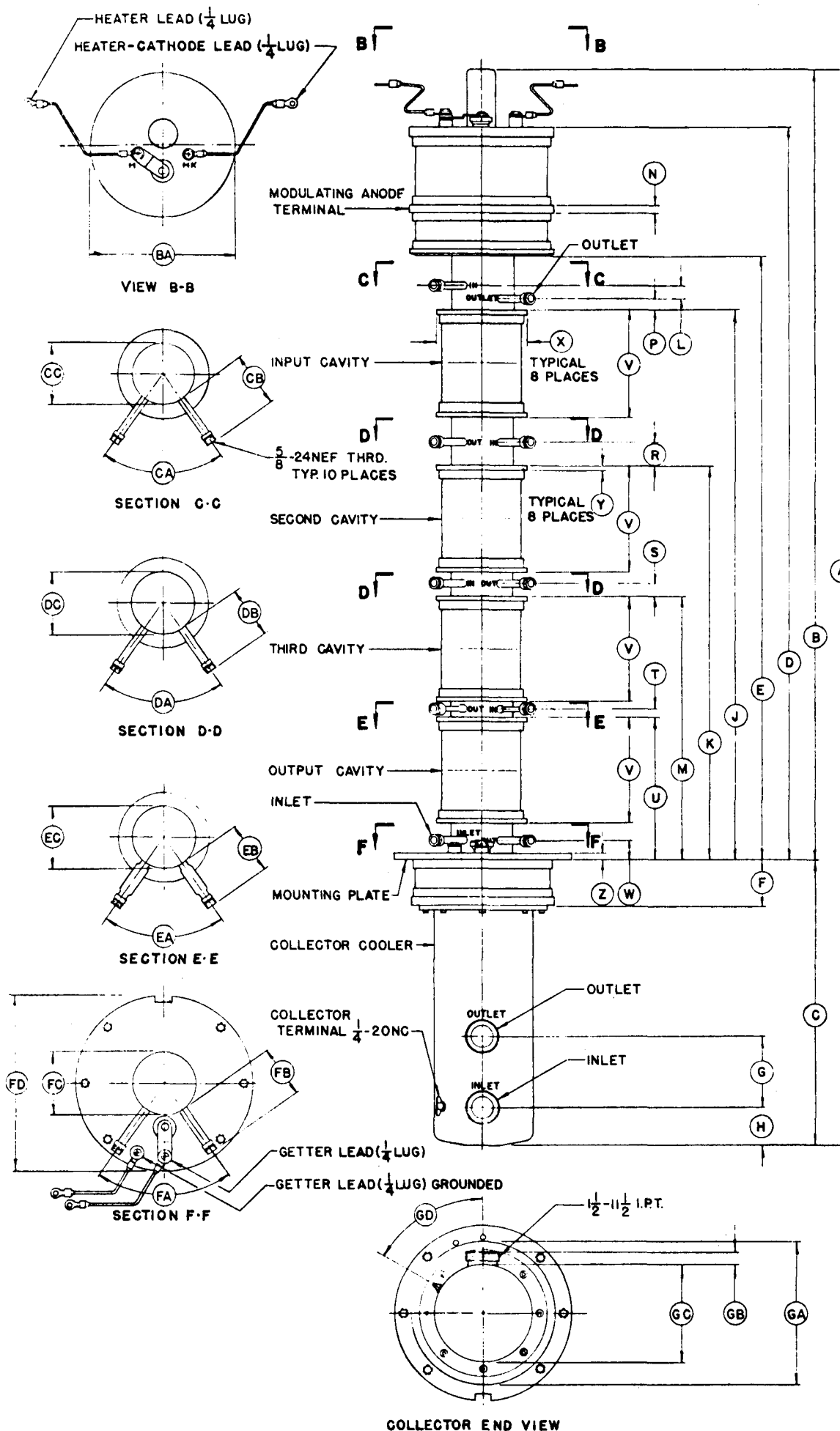
4KM100LA KLYSTRON
