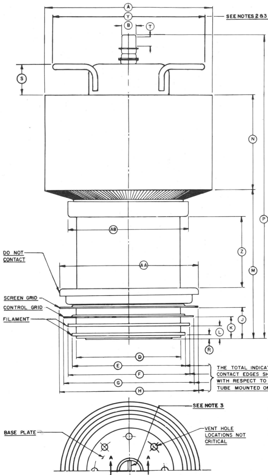
SECTION A-A
