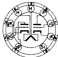
BOTTOM VIEW MINIATURE BUTT 9 PIN NOVAL 9AU
