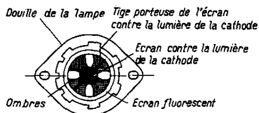
Vue en plan du trèfle cathodique et de son support. La tige qui porte la coupelle donne la position de la croix.
