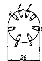
Disposition des électrodes et connexions du culot.
