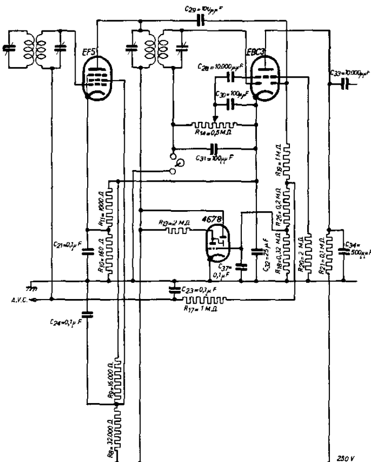
Montage du tréfle cathodique 4678 dans un récepteur sur alternatif avec réglage automatique différé. La tension régulatrice appliquée aux grilles des lampes réglées est réduite au moyen du diviseur de tension R_{18} pour le tréfle cathodique afin d'obtenir une plage de réglage correcte pour ce dernier.
