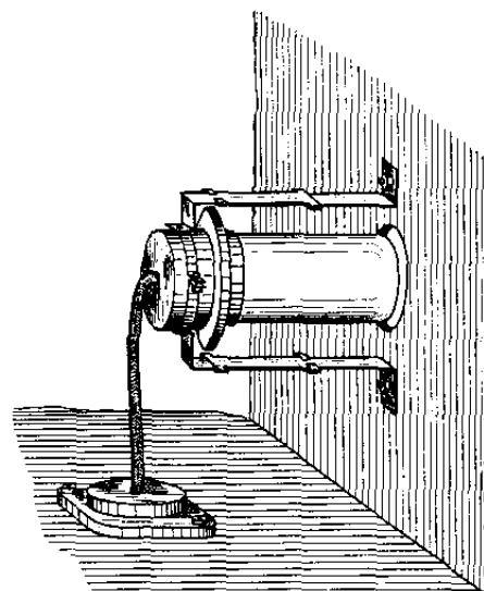
Exemple de montage du tréfle cathodique dans un récepteur. Pour interchanger ce tube on fait glisser le support en arrière.
