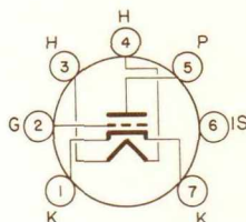
BOTTOM VIEW JEDEC 7 FP
