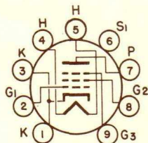
BASING DIAGRAM JEDEC 9AQ BOTTOM VIEW
