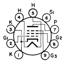
BOTTOM VIEW BASING DIAGRAM JEDEC 9AQ
