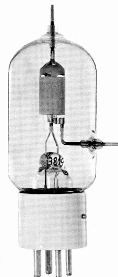
EIMAC HR-3
