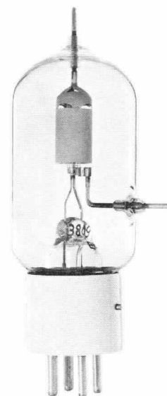
EIMAC HR-3
