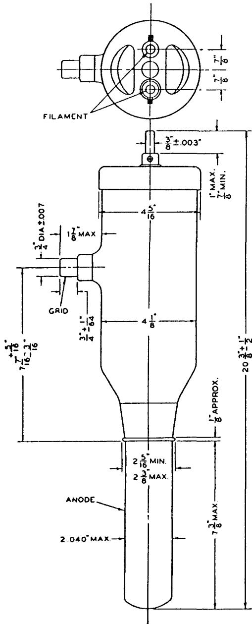
DIMENSIONS — ML-343A
