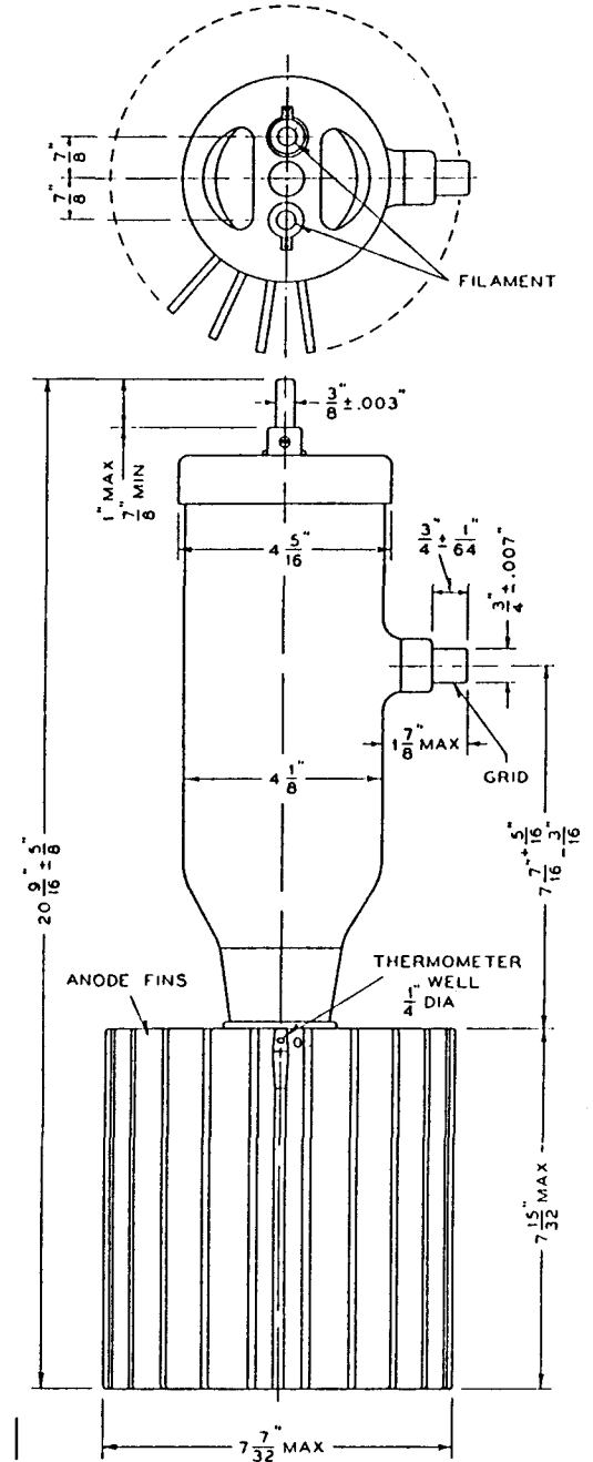
DIMENSIONS — ML-343AA
