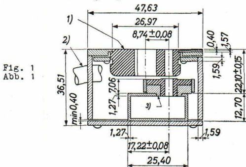
Cross-section of the mount Coupe transversale du montage Querschnitt der Halterung
