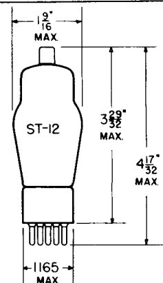
2B7, 6B7
