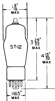
6B8G
