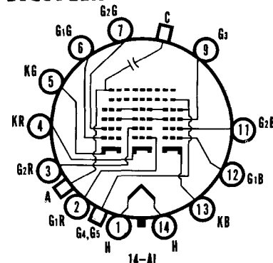
21FBP22 21FJP22 21FKP22
