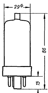
Kolbenabmessungen
