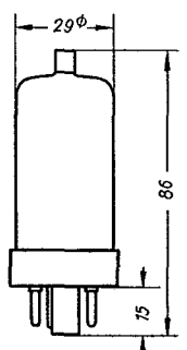
Kolbenabmessungen
